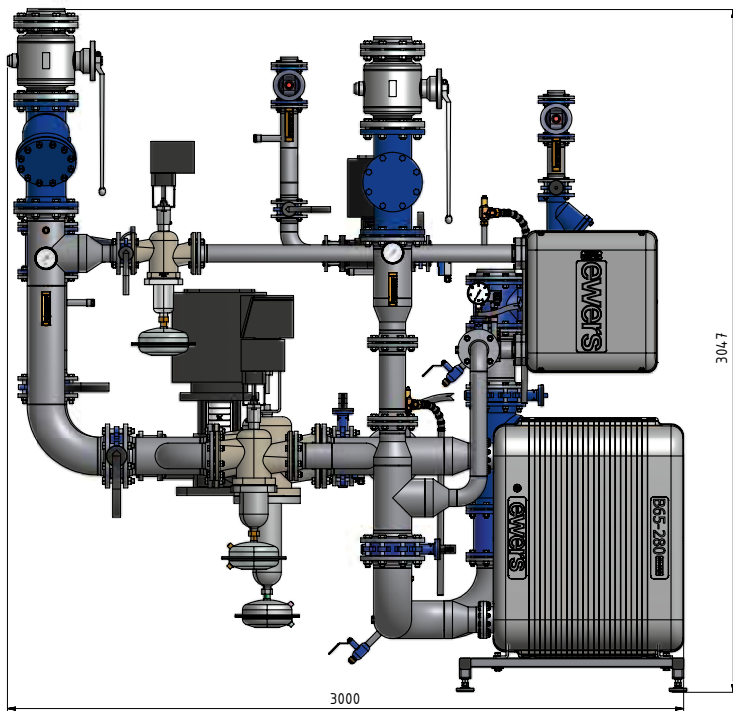
Zeichnung der Fernwärmewärme Übergabestation
