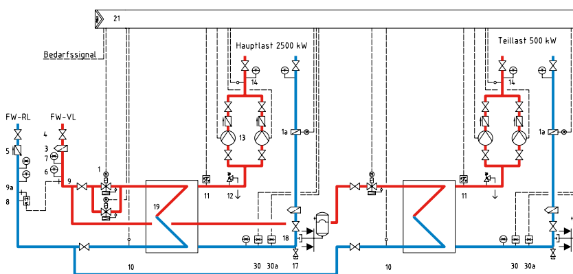
Hydraulische Darstellung
