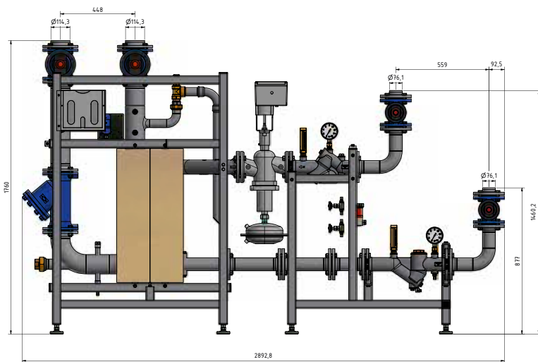
Technische Zeichnung
