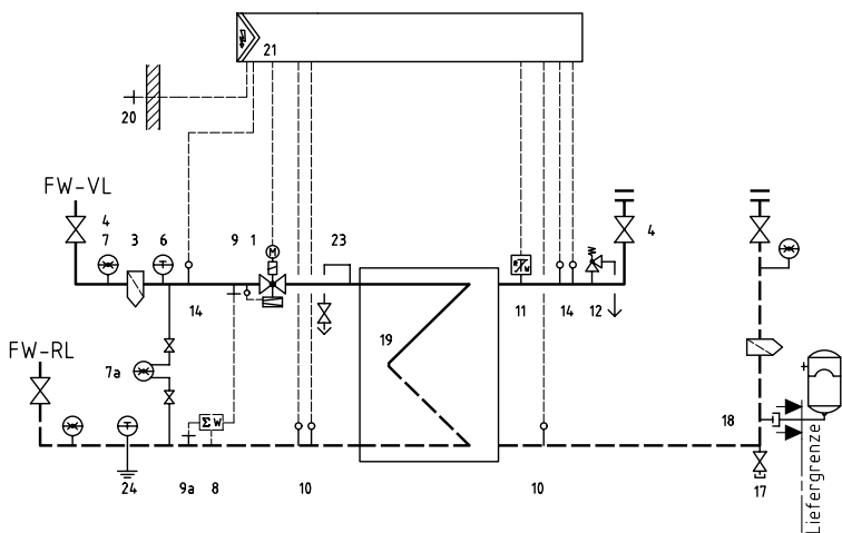
Hydraulische Darstellung
